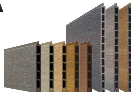
PROFIL OGRODZENIOWY WPC PREMIUM 21 x 160 / 310 x 1780 mm (DB 150/300 mm) Ciemnoszary Art. 2315 / 2318 Jasnoszary Art. 2316 / 2467 Czerwony cedr Art.2777 Teak Art. 2317 / 2473 Ipé Art.2314
