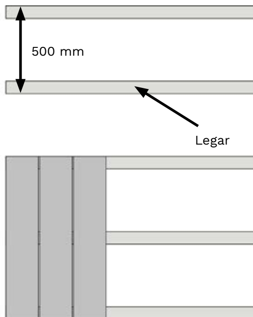
Montaż pionowy
